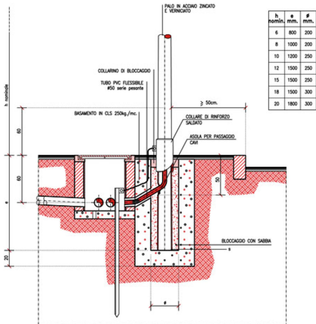
PARTICOLARE MESSA IN OPERA E FONDAZIONE PALO E POZZETTO DI COLLEGAMENTO ILLUMINAZIONE PUBBLICA
