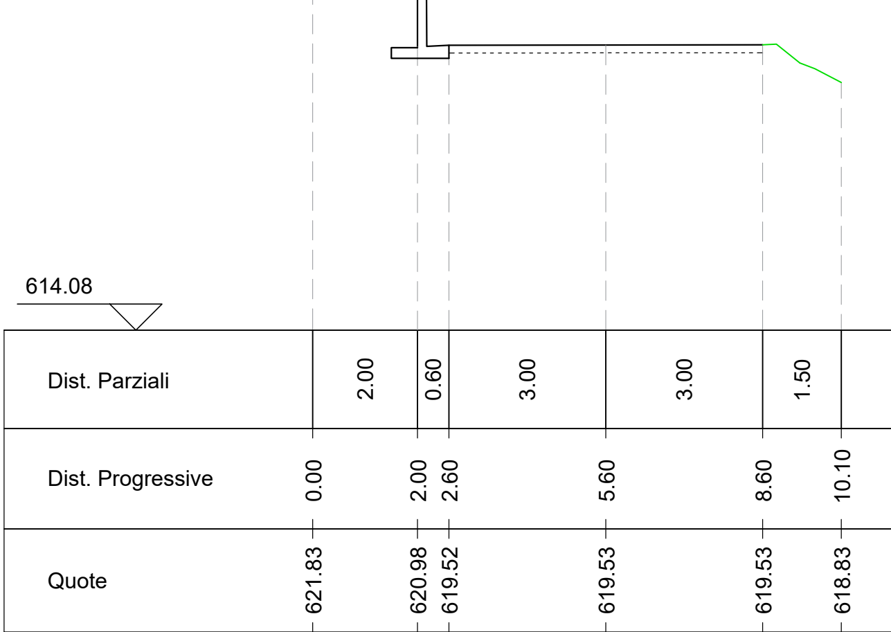
Sezione B1 Altezze: 1:100 Lunghezze: 1:100
