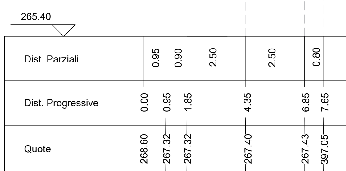
Sezione C9 Altezze: 1:100 Lunghezze: 1:00
