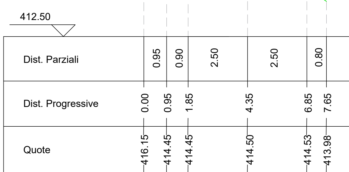
Sezione C7 Altezze: 1:100 Lunghezze: 1:00
