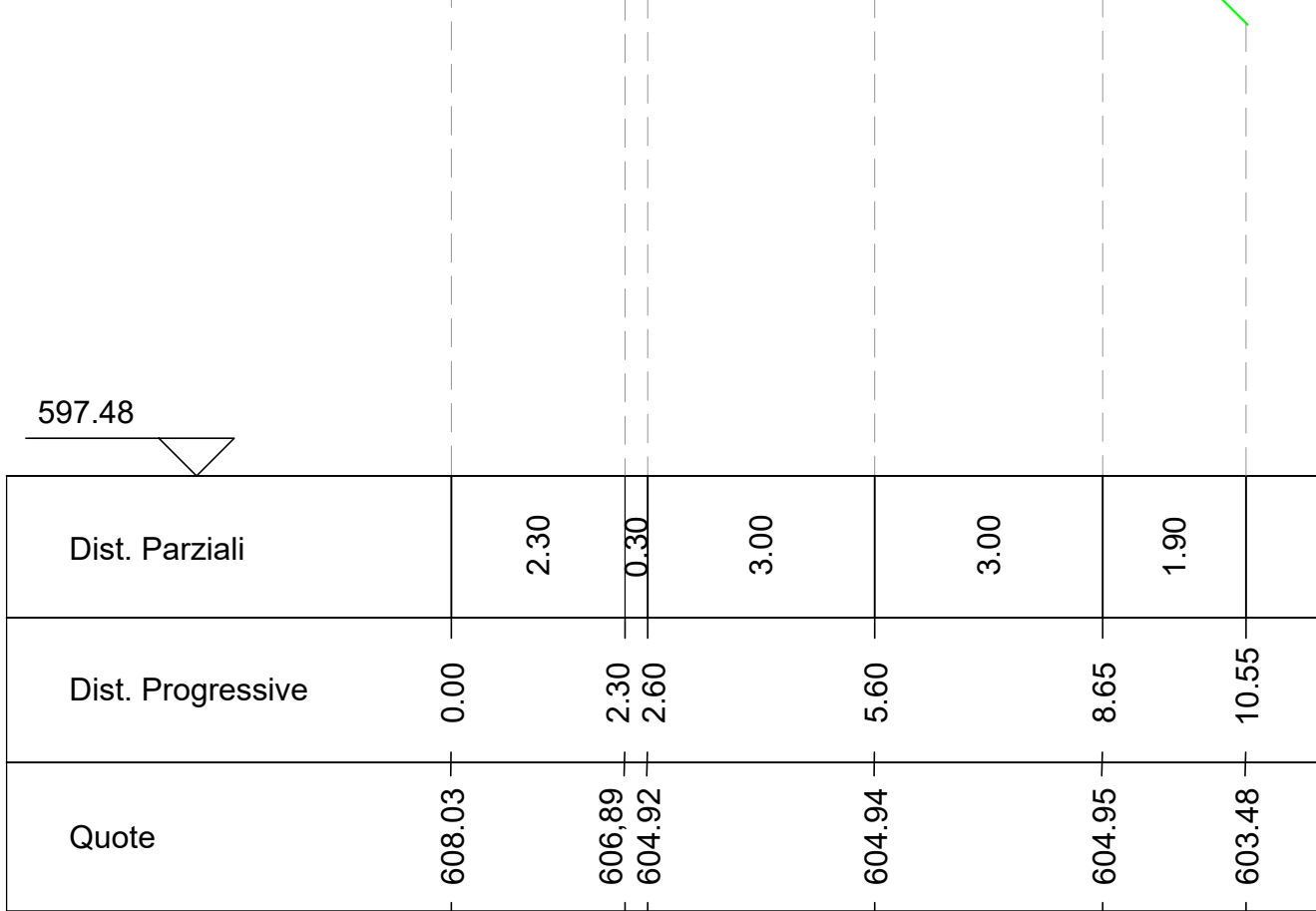
Sezione B2 Altezze: 1:100 Lunghezze: 1:100
