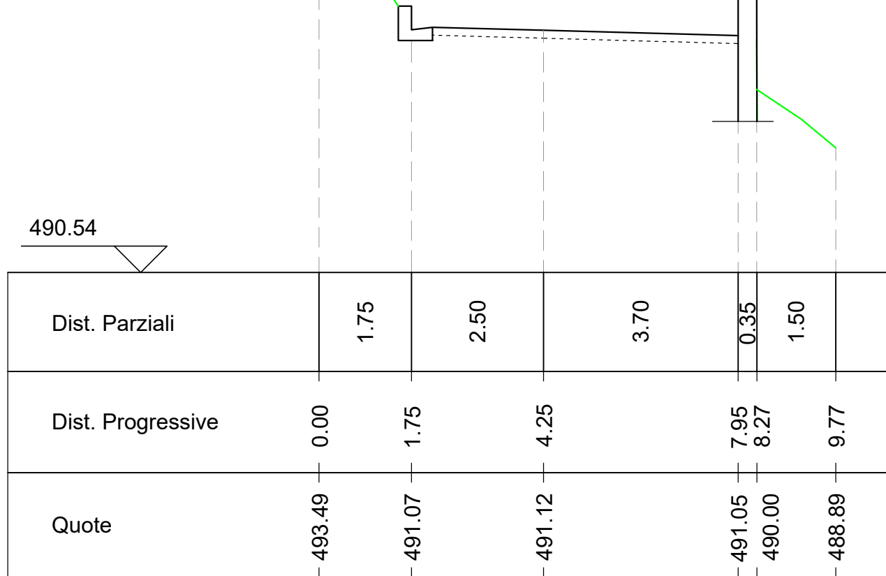
Sezione C3 Altezze: 1:100 Lunghezze: 1:00
