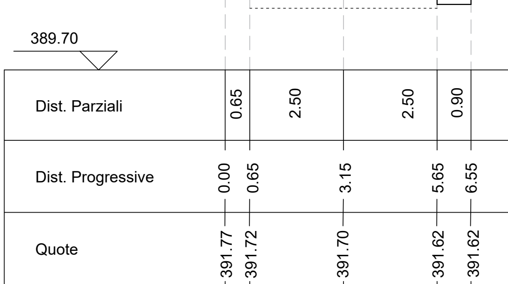
Sezione C11 Altezze: 1:100 Lunghezze: 1:00
