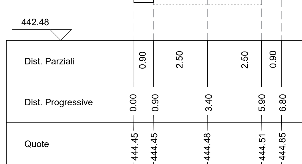
Sezione C10 Altezze: 1:100 Lunghezze: 1:00
