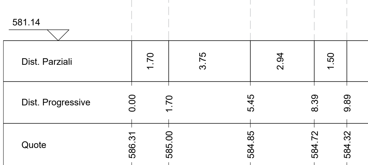
Sezione C8 Altezze: 1:100 Lunghezze: 1:00
