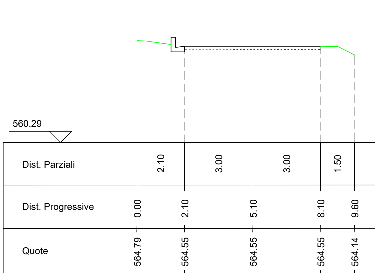
Sezione B3 Altezze: 1:100 Lunghezze: 1:100
