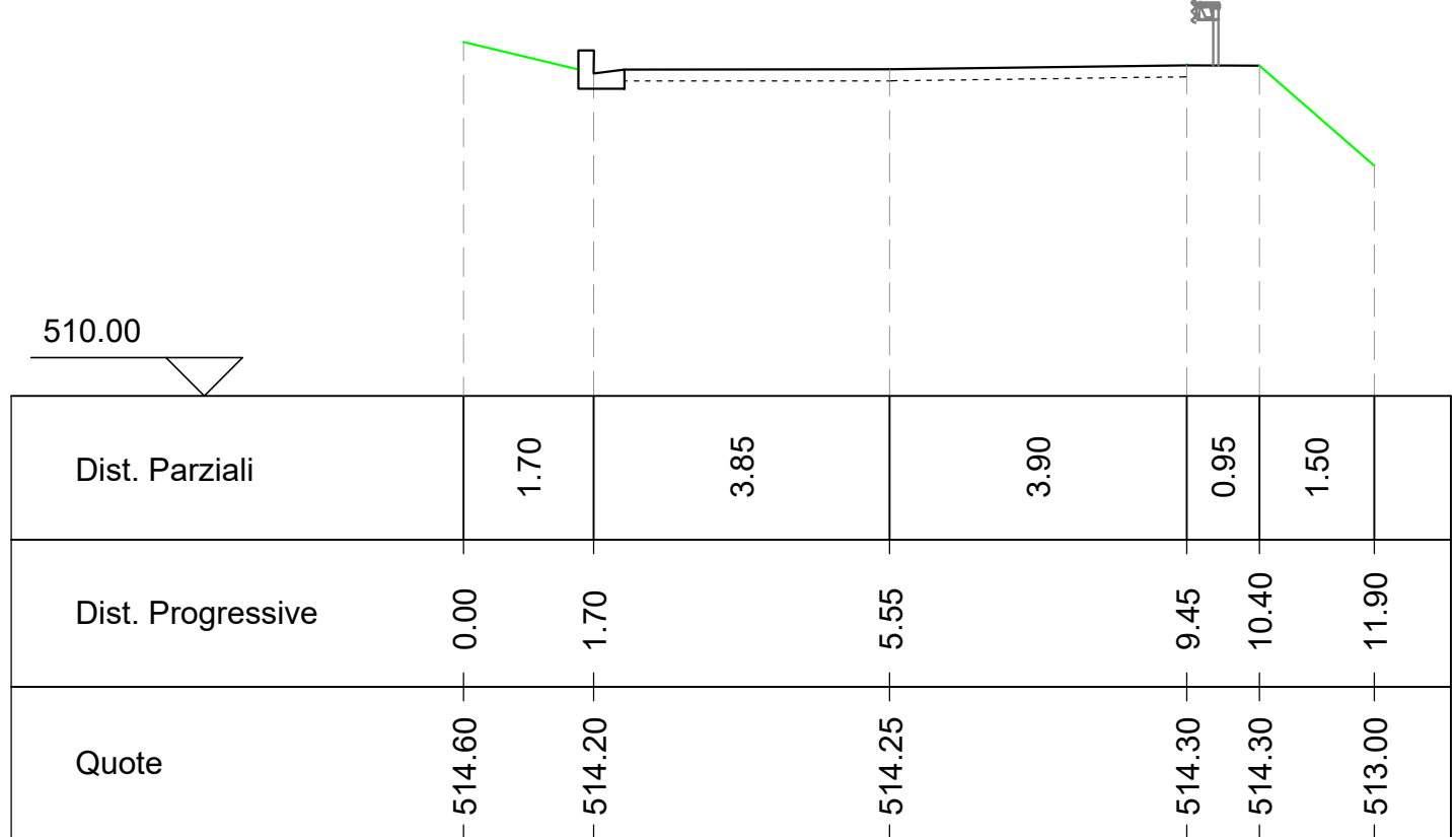
Sezione B6 Altezze: 1:100 Lunghezze: 1:100
