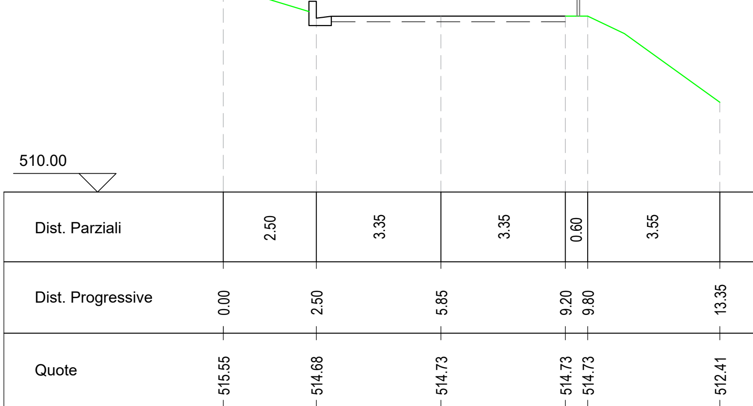
Sezione C1 Altezze: 1:100 Lunghezze: 1:00
