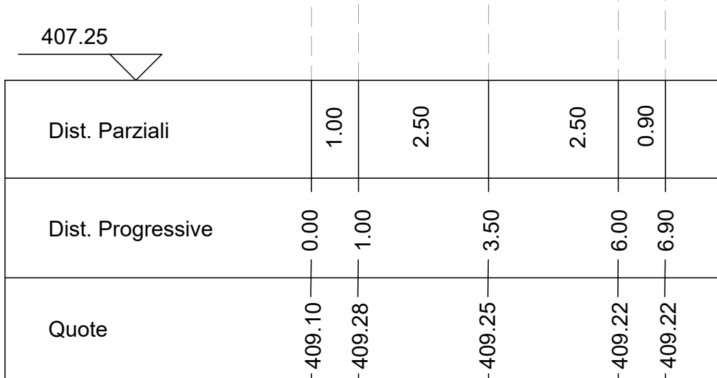
Sezione C8 Altezze: 1:100 Lunghezze: 1:00
