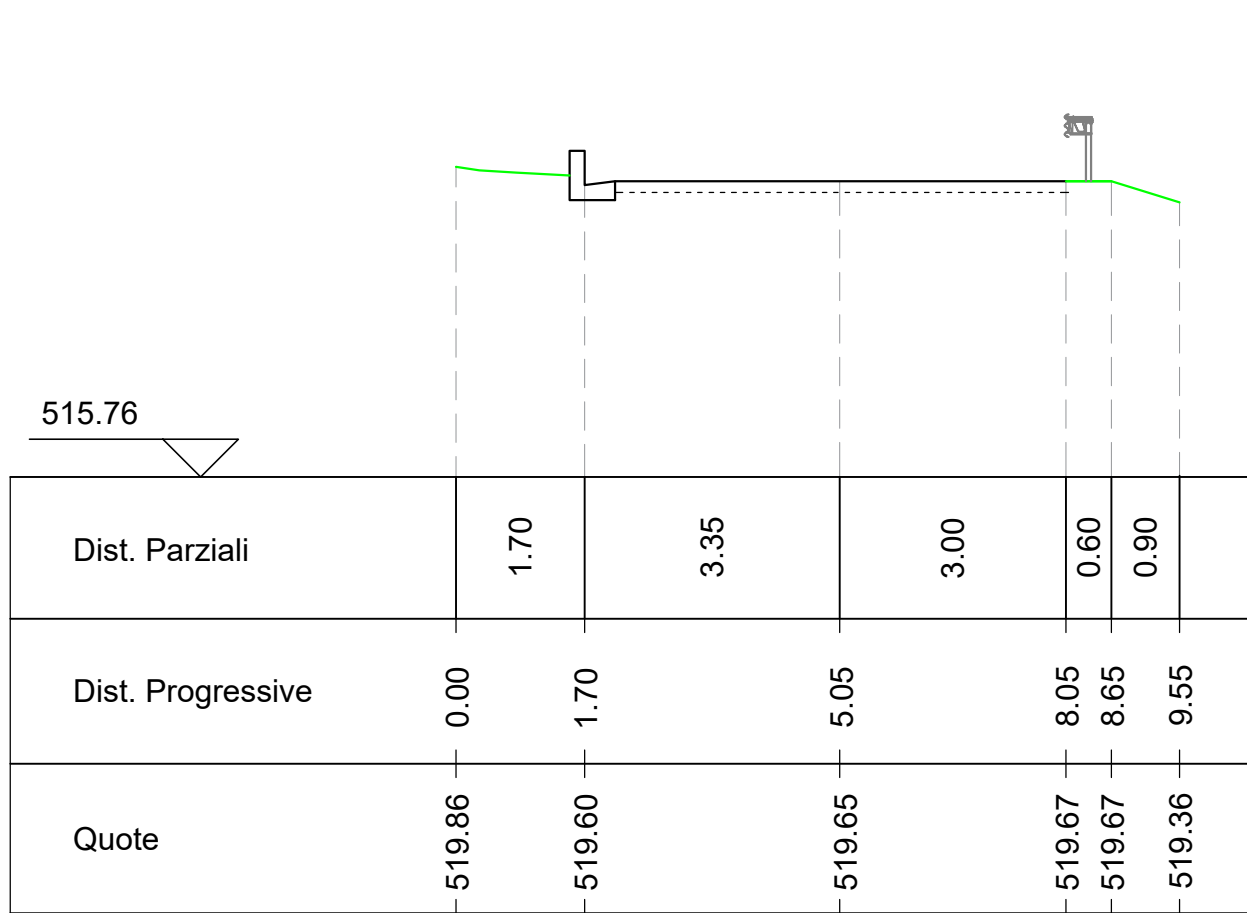
Sezione B4 Altezze: 1:100 Lunghezze: 1:100
