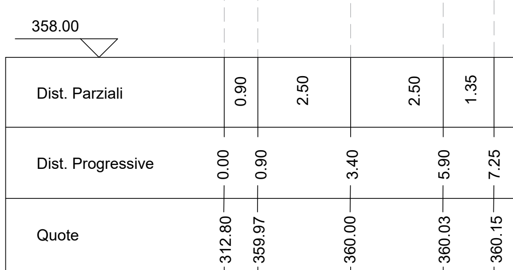
Sezione C5 Altezze: 1:100 Lunghezze: 1:00
