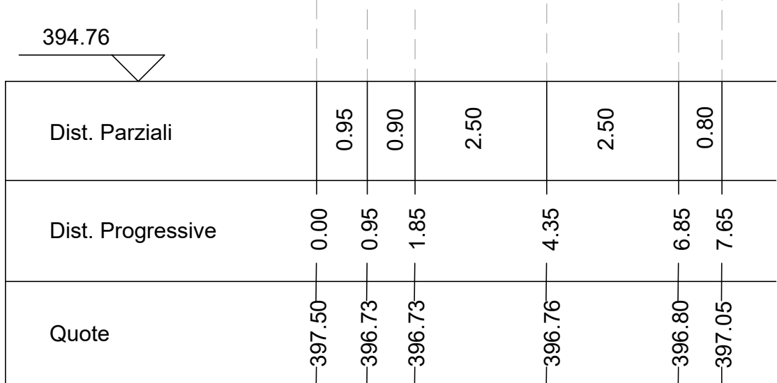
Sezione C6 Altezze: 1:100 Lunghezze: 1:00
