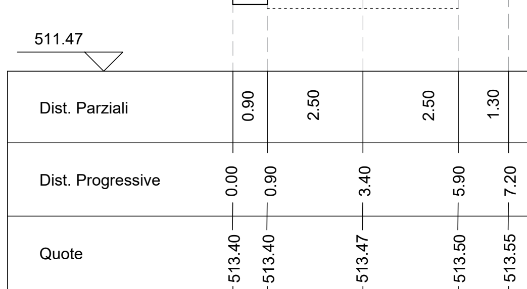
Sezione C9 Altezze: 1:100 Lunghezze: 1:00
