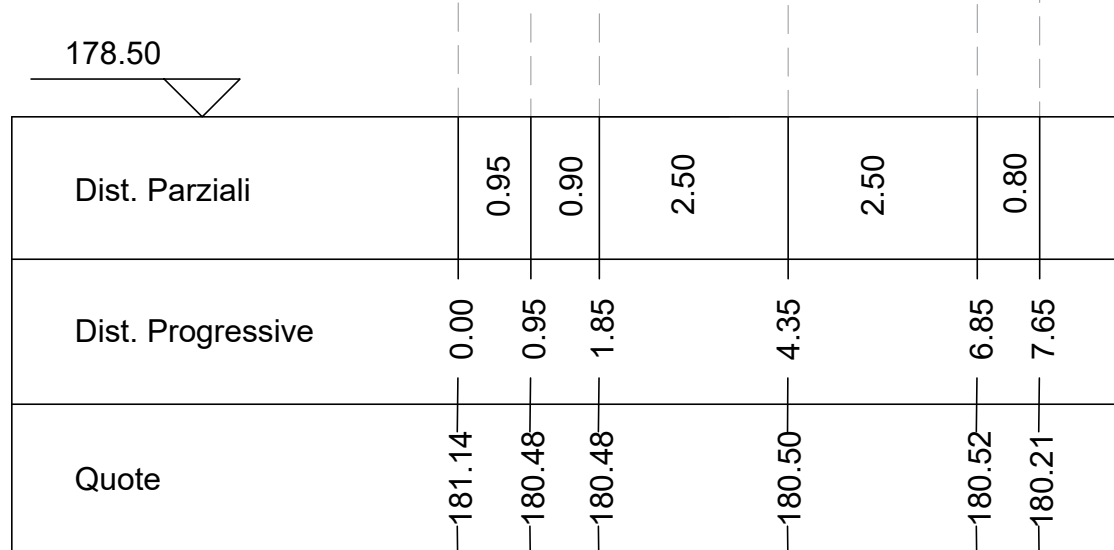
Sezione C10 Altezze: 1:100 Lunghezze: 1:00
