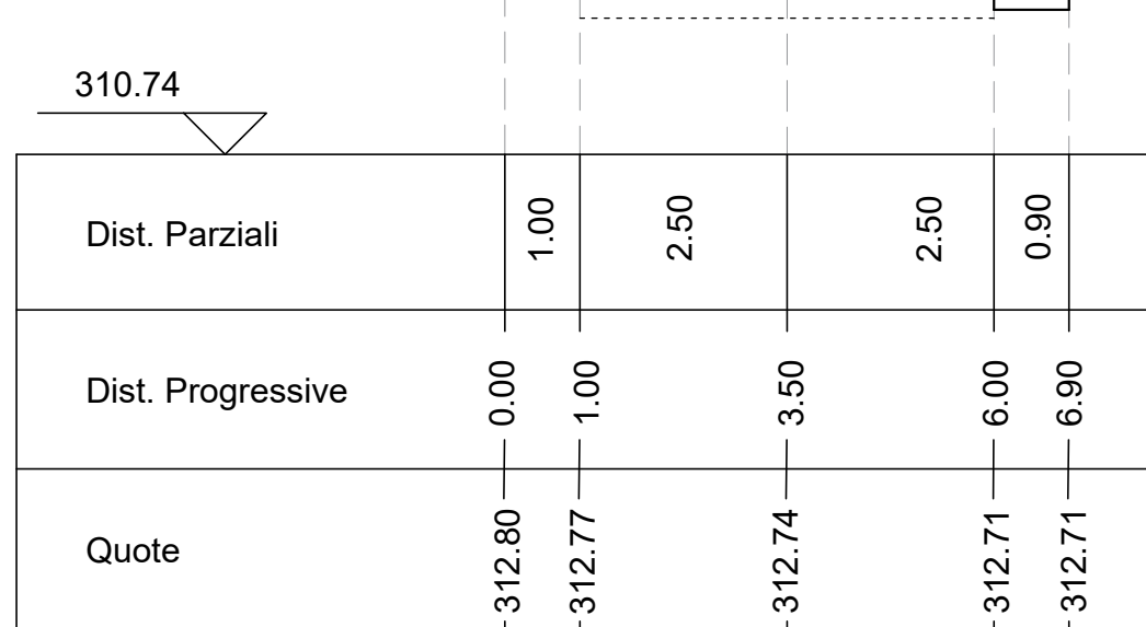
Sezione C4 Altezze: 1:100 Lunghezze: 1:00
