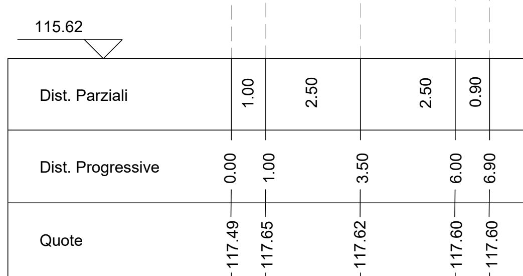
Sezione C11 Altezze: 1:100 Lunghezze: 1:00
