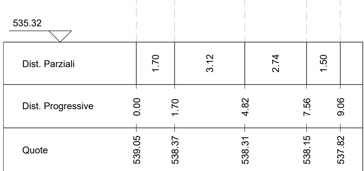
Sezione C5 Altezze: 1:100 Lunghezze: 1:00
