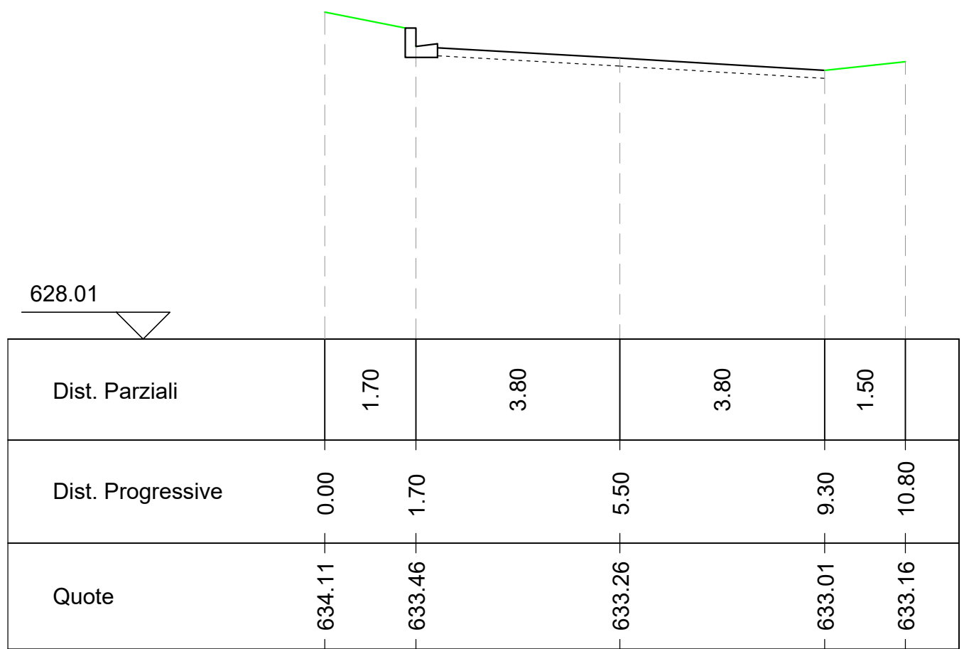
Sezione A6 Altezze: 1:100 Lunghezze: 1:100
