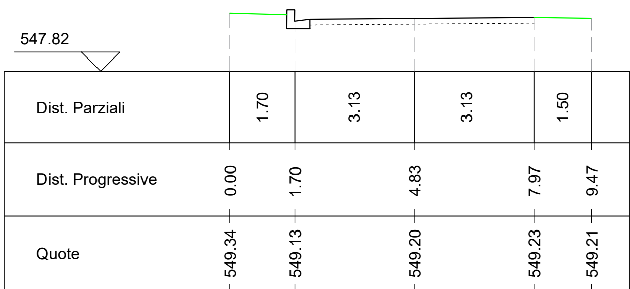
Sezione C6 Altezze: 1:100 Lunghezze: 1:00
