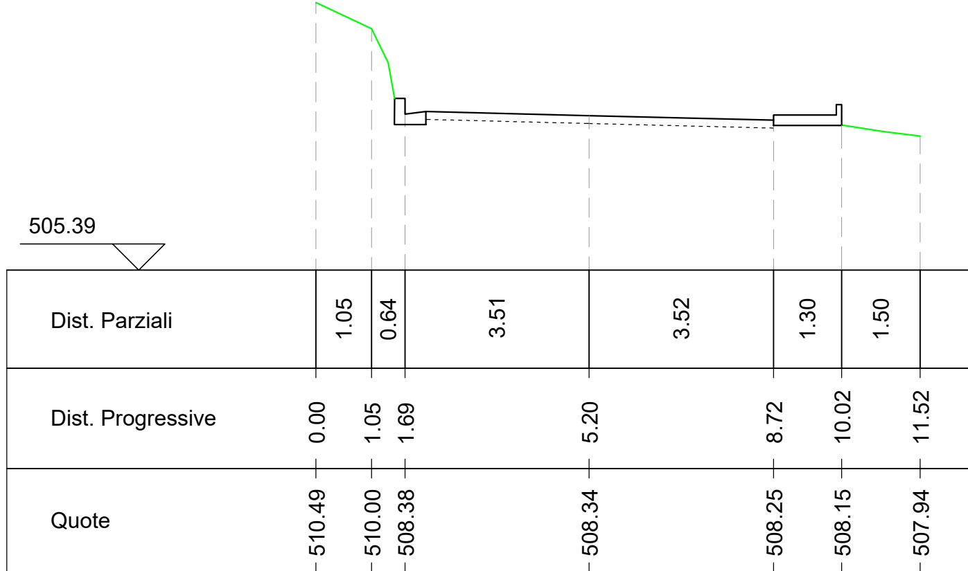
Sezione C4 Altezze: 1:100 Lunghezze: 1:00
